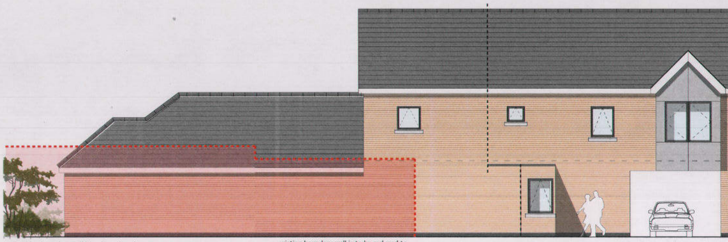
elevation 1
